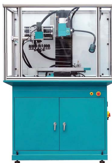
iKX 3 S (Siemens)
