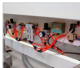
▶ Regulace stlačeného vzduchu
