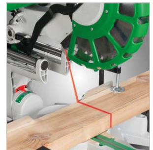
▶ Laserový ukazatel k vyznačení linie řezu
