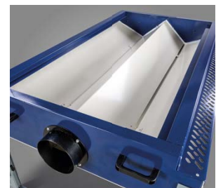
▶ Třichtýřový vzduchový kanál k odsávacímu nátrubku pro rovnoměrný sací výkon
