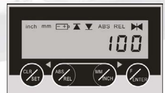
Obr.: Délkové odměřování LMS 10 na válečkové trati MSR 4.
