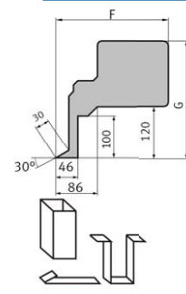
Horní lišta MSBM SH
