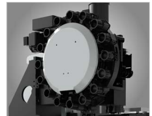
Bubnový výměník nástrojů s ramenem (F 110 HSC)
